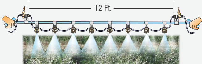
स्प्रे बूम (८ नोजलस)
